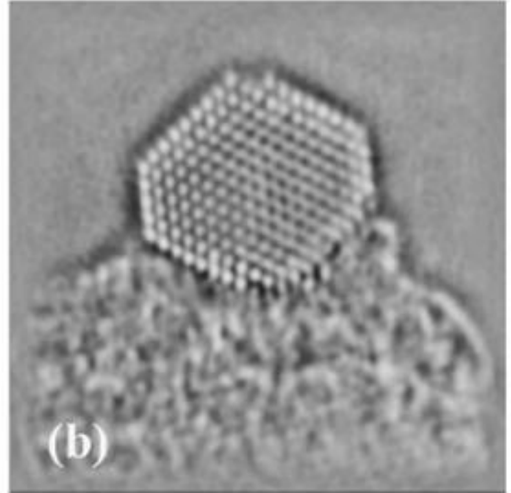
TEM s korekcí aberací
